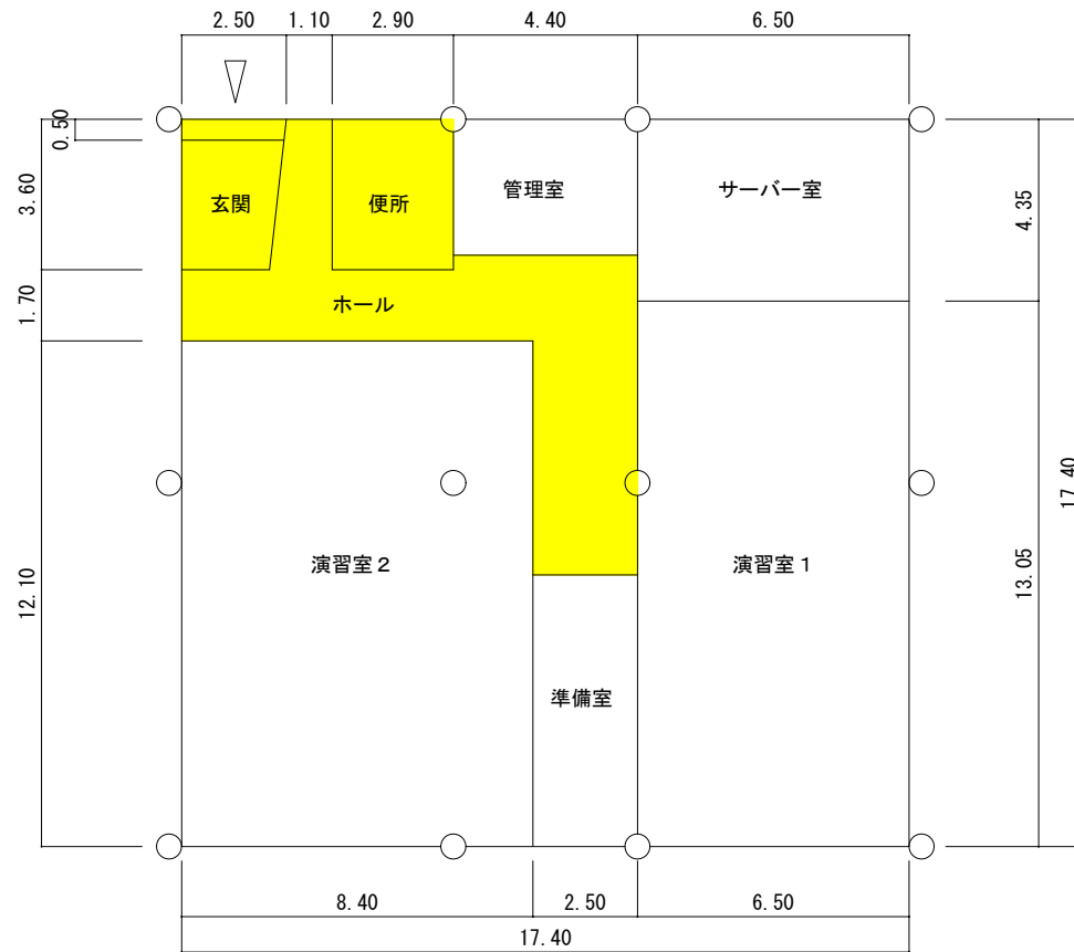
平面図 S=1/200 301㎡
