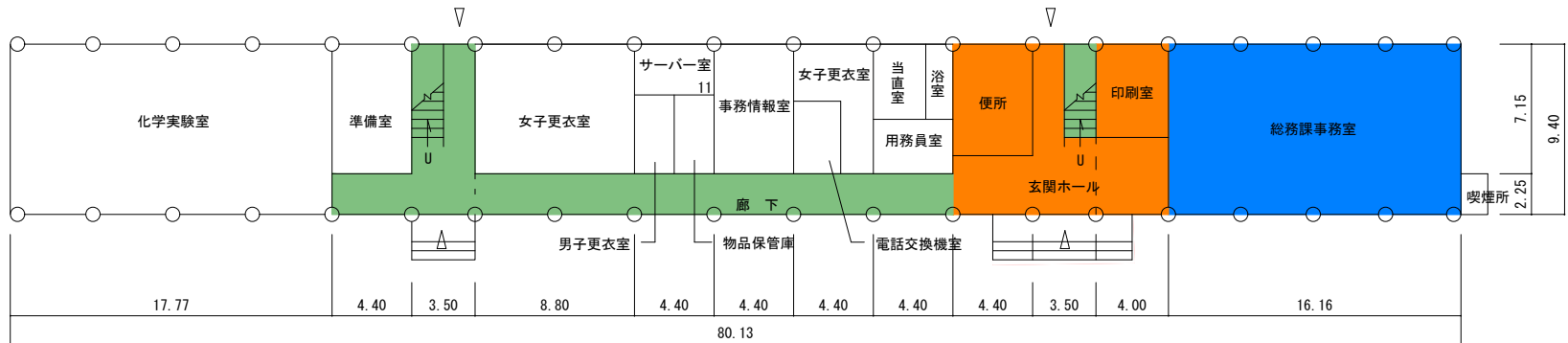
1階 平面図 S=1/400 753㎡
