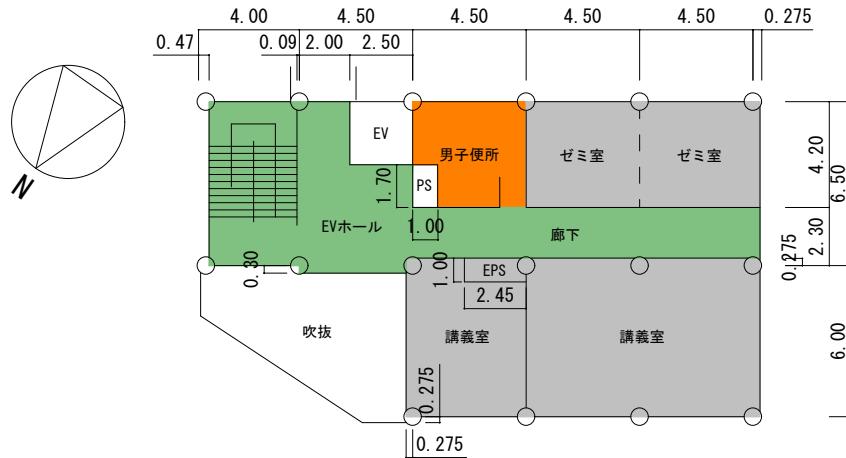
2階 平面図 S=1/300 228㎡
