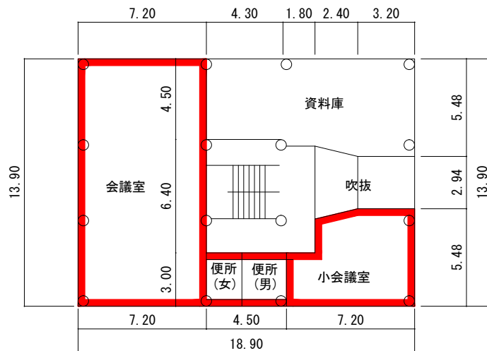
2階 平面図 S=1/300 245㎡
