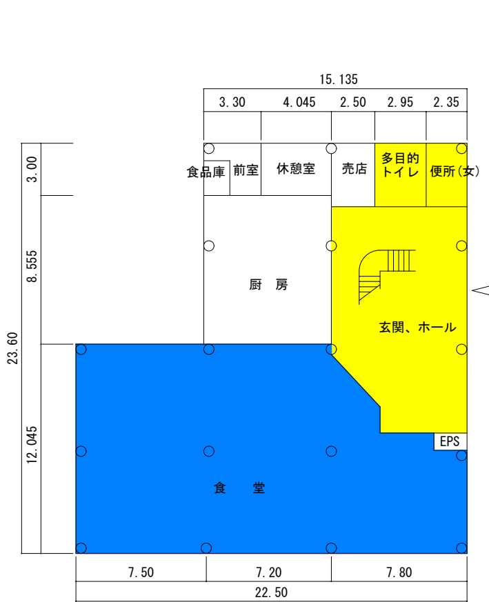
1階 平面図 S=1/300 440㎡
