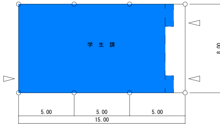
平面図 S=1/200 120㎡
