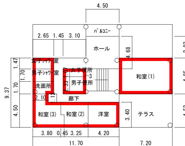
3階 平面図 S=1/300 157㎡
