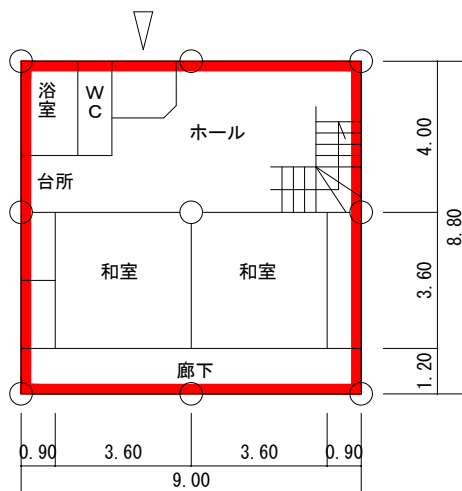
1階平面図 S=1/200 79㎡
