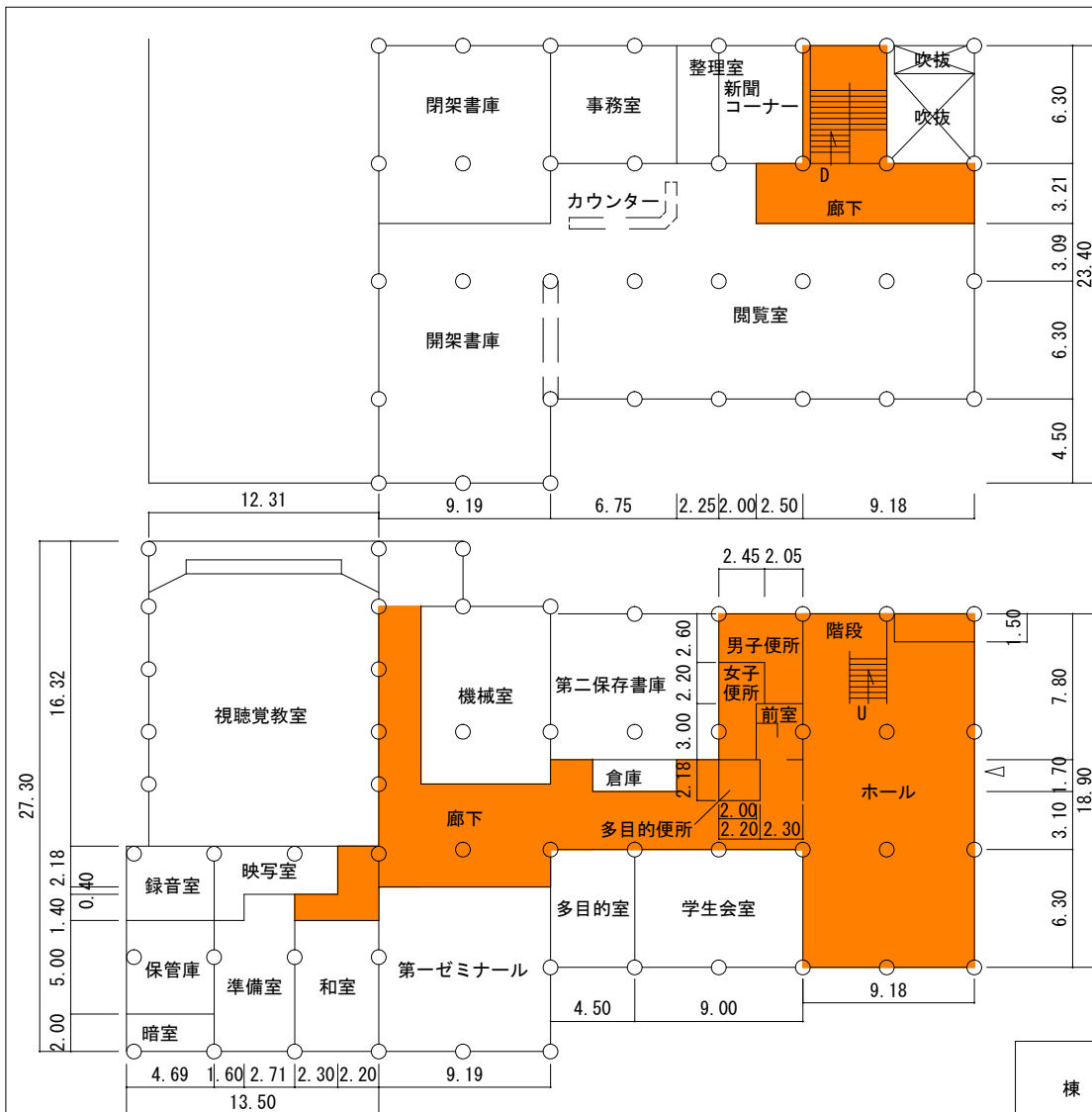
2階 平面図 S=1/400 604㎡
