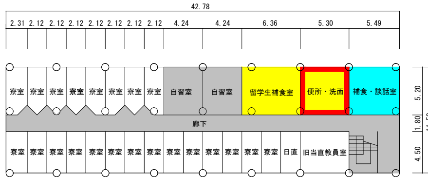
3階 平面図 S=1/400 492㎡
