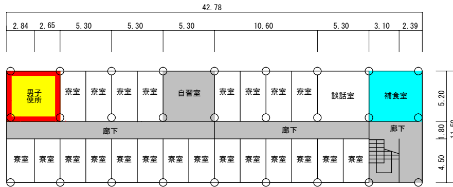
2階 平面図 S=1/400 492㎡
