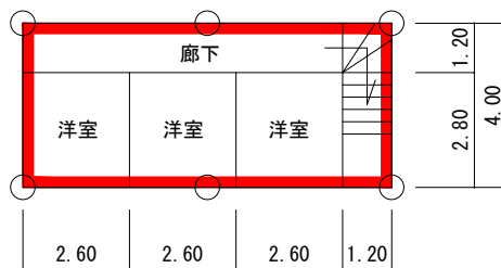
2階平面図 S=1/200 36㎡
