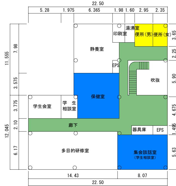
2階 平面図 S=1/300 440㎡
