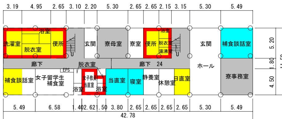
1階 平面図 S=1/400 492㎡
