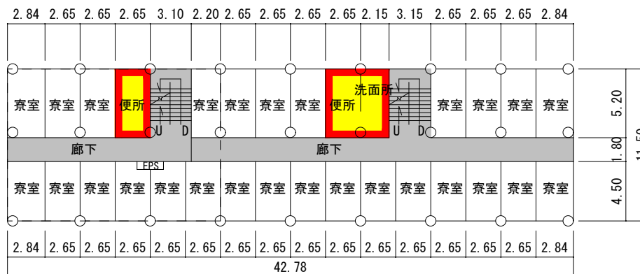
2~4階 平面図 S=1/400 492㎡
