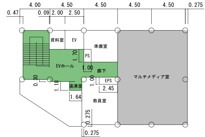
3階 平面図 S=1/300 230㎡
