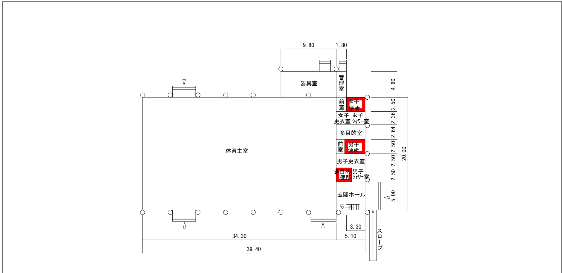
平面図 S=1/400 841m 2
