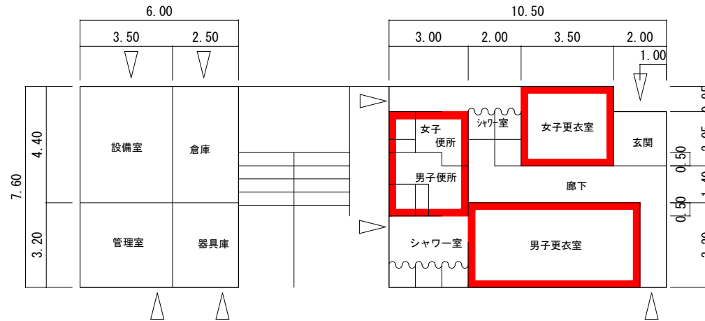
平面図 S=1/200 124㎡
