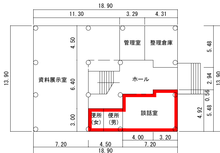
1階 平面図 S=1/300 258㎡
