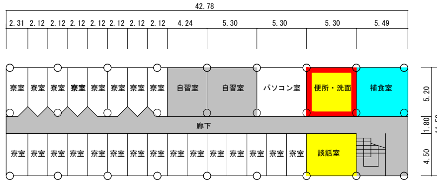
4階 平面図 S=1/400 492㎡
