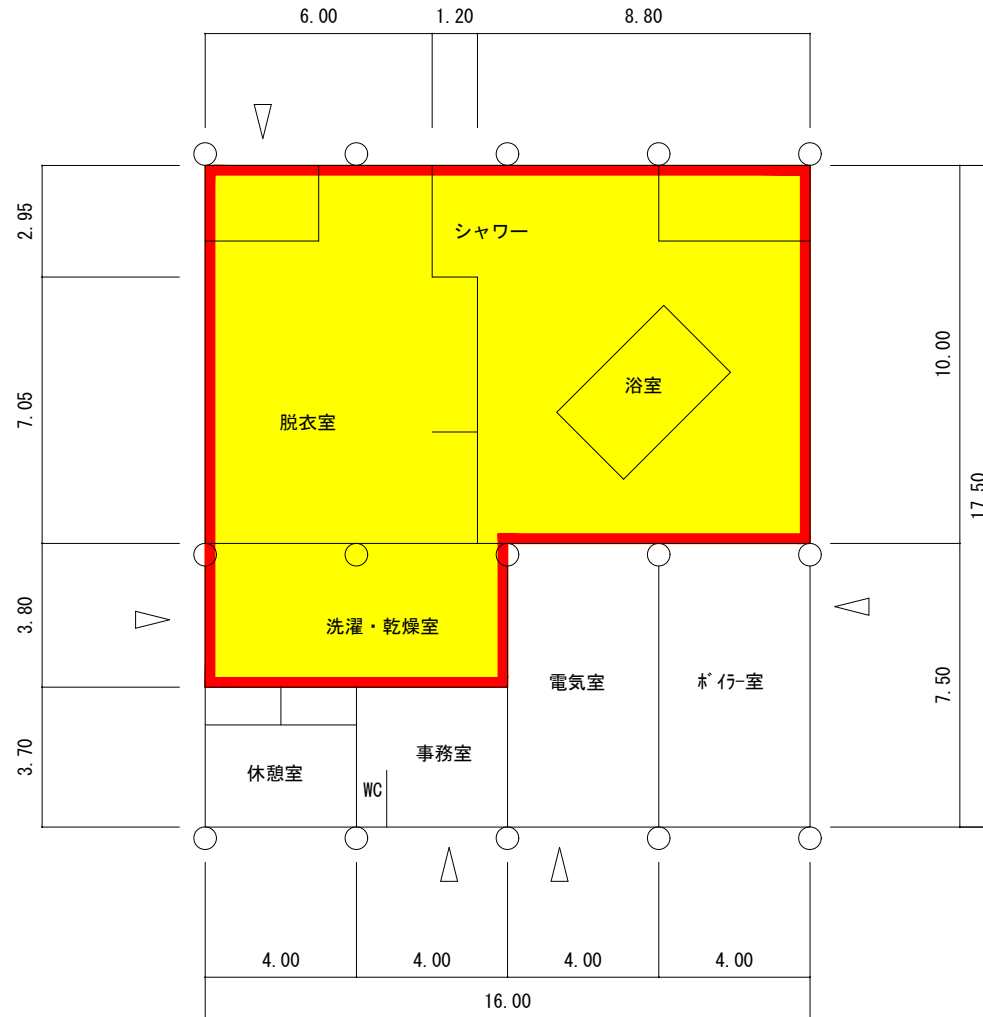
平面図 S=1/200 280㎡
