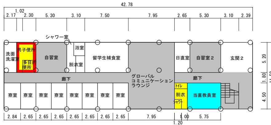
1階 平面図 S=1/400 492㎡
