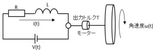
図1 モータのモデル
